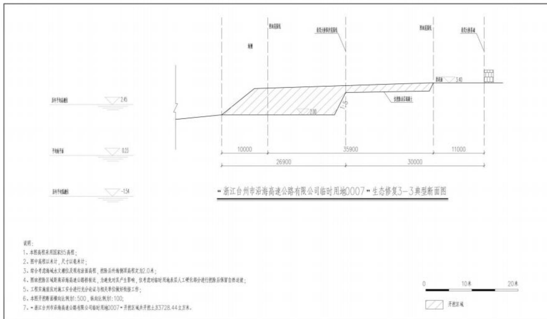
图 8 典型断面图 3-3
