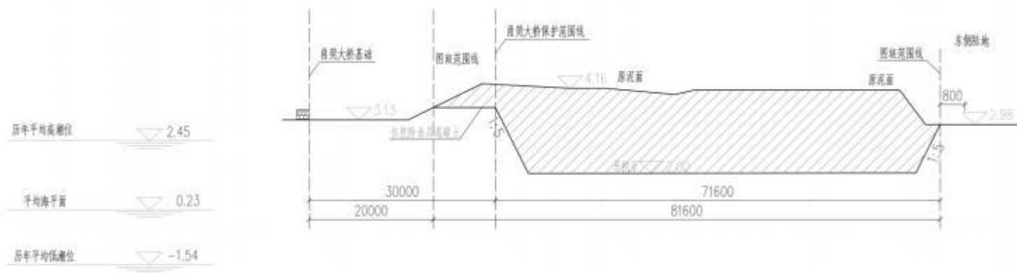
“浙江台州市沿海高速公路有限公司临时用地0008、0009”生态修复2-2典型断面图
