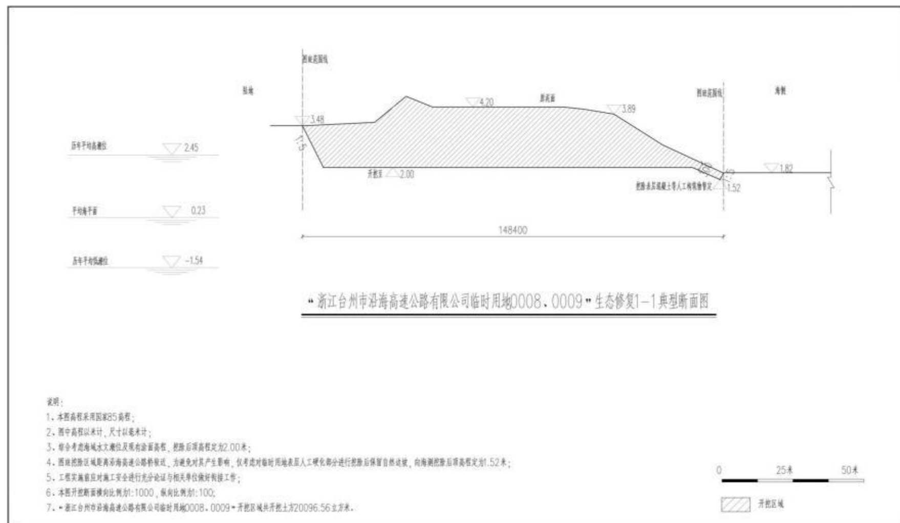
图 6 典型断面图 1-1
